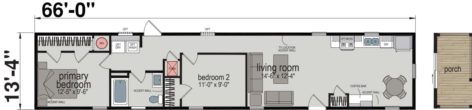
Optional Porch
